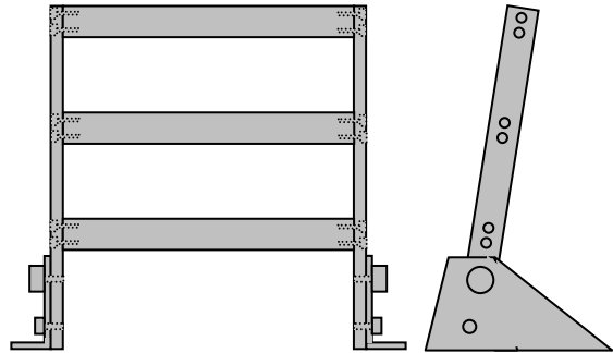
Vues frontales du Support
